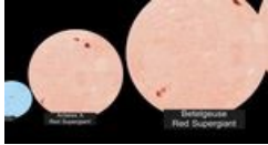
Comparación de los tamaños de las estrellas
